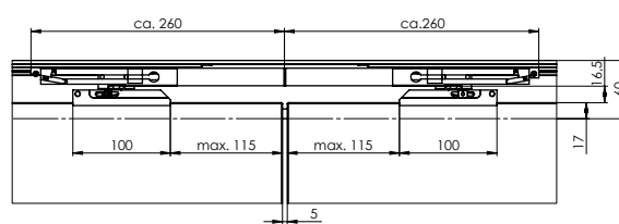
tuerdaempfer zweifluegelig
